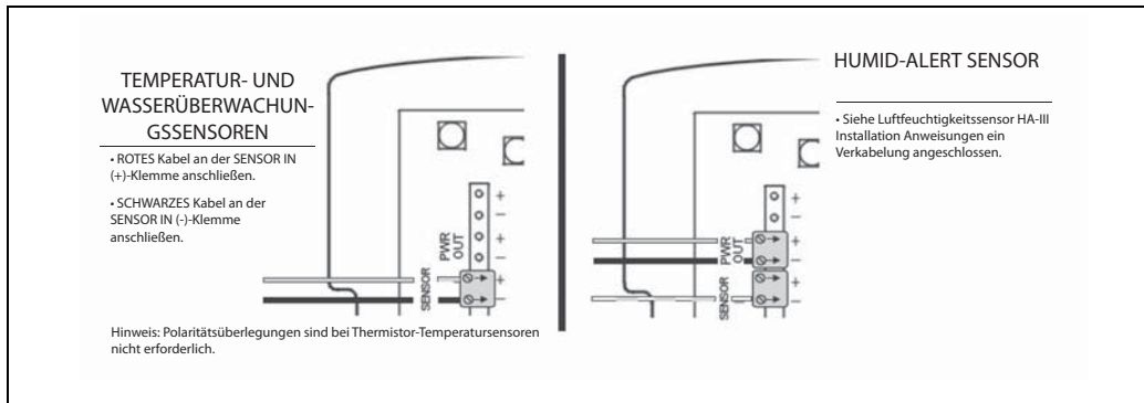
Abbildung 7. Sensoranschlüsse des EA200 bzw. EA400
