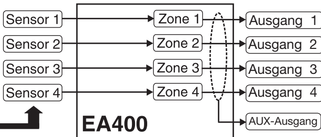
Abbildung 3. EA400-Funktionsdiagramm
