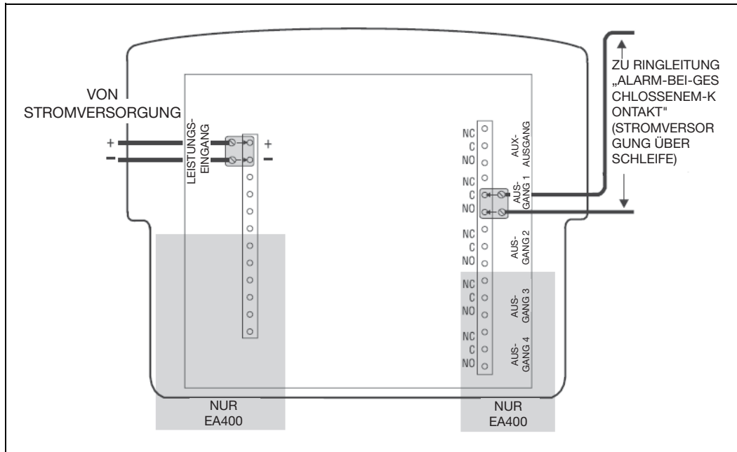
Abbildung 8. Typische Alarmschleifenverkabelung (externe Stromversorgung)
