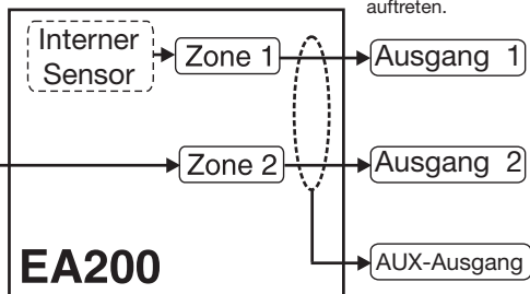
Abbildung 2. EA200-Funktionsdiagramm
