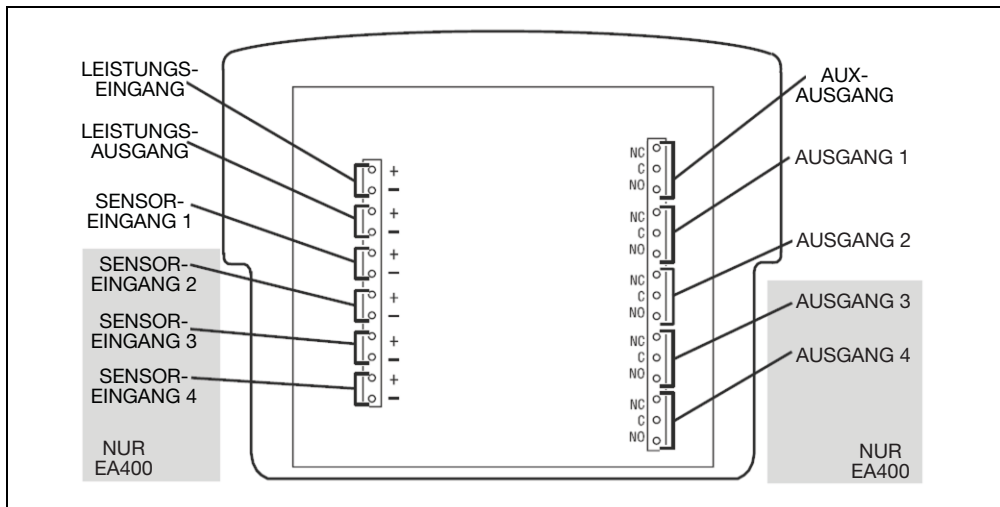
Abbildung 6. Anschlüsse des EA200 bzw. EA400
