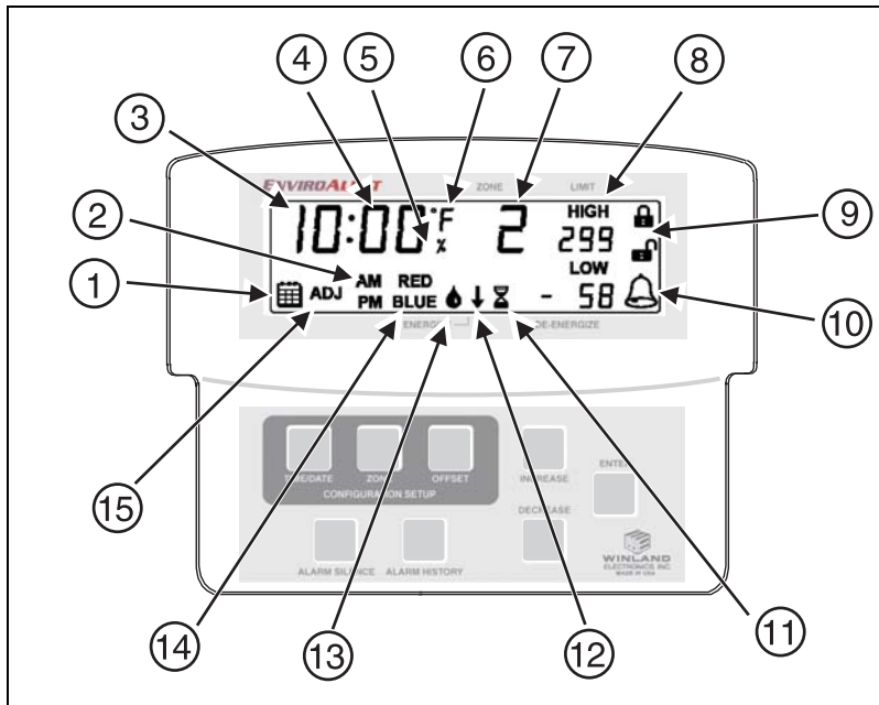
Abbildung 4. EA200 / EA400 Anzeige und Symbole
