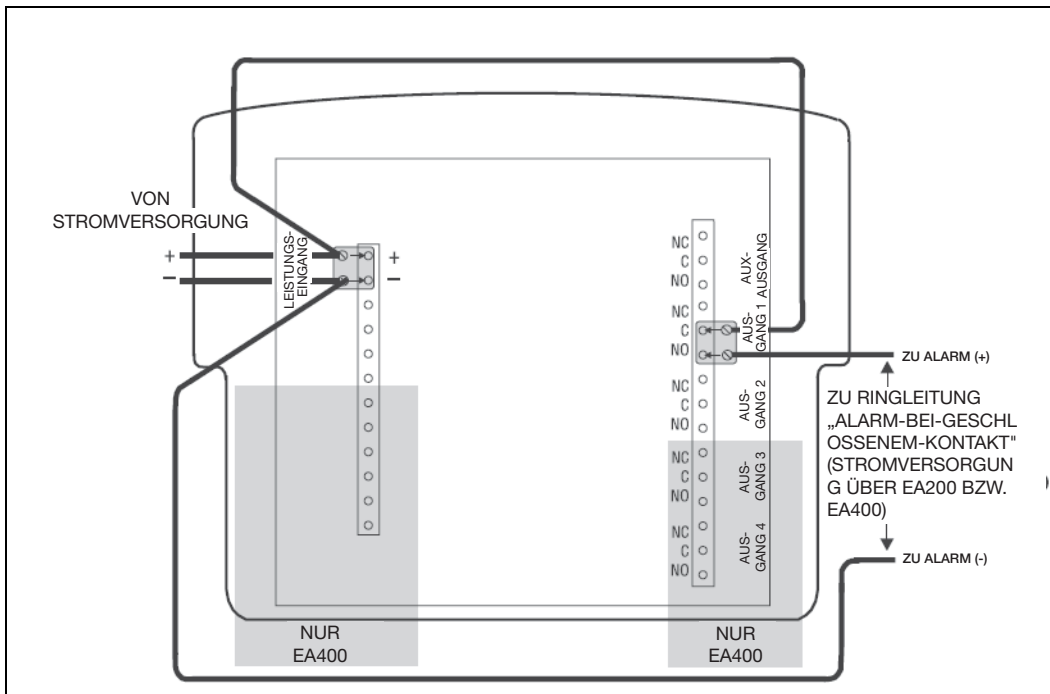
Abbildung 9. Typische Alarmschleifenverkabelung (eigene Stromversorgung)
